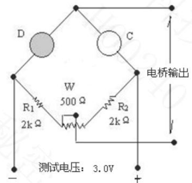
图 2：基本测试电路
