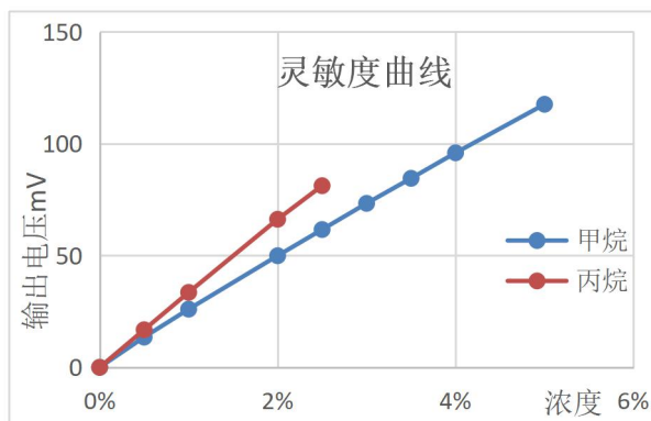
图3：灵敏度曲线
